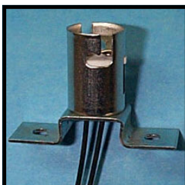
Douille baïonnette 2 contacts Fil amiante
